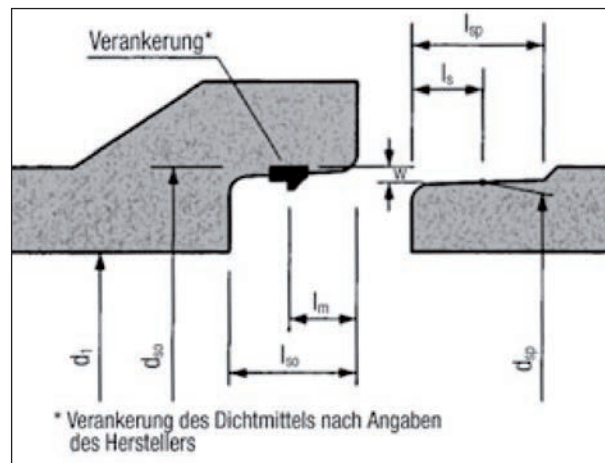
Bild 1: Gleitringdichtung werkseitig fest in der Muffe eingebaut (Beispiel)
