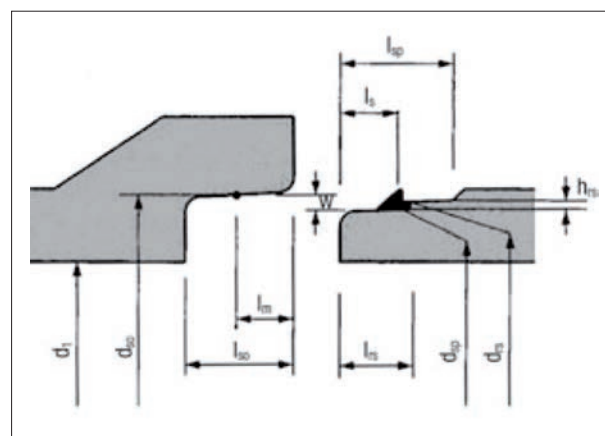
Bild 3: Gleitringdichtung für Stufenausbildung (Beispiel)
