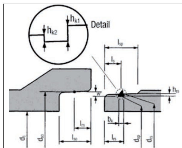
Bild 2: Gleitringdichtung für Kammerausbildung (Beispiel)
