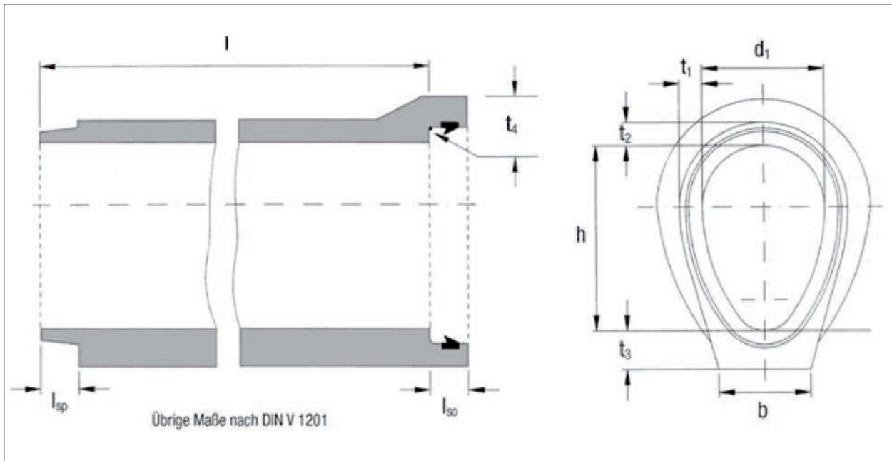
Bild 4: FBS-Rohr mit Eiquerschnitt und werkseitig fest in der Muffe eingebauter Gleitring-Dichtung
